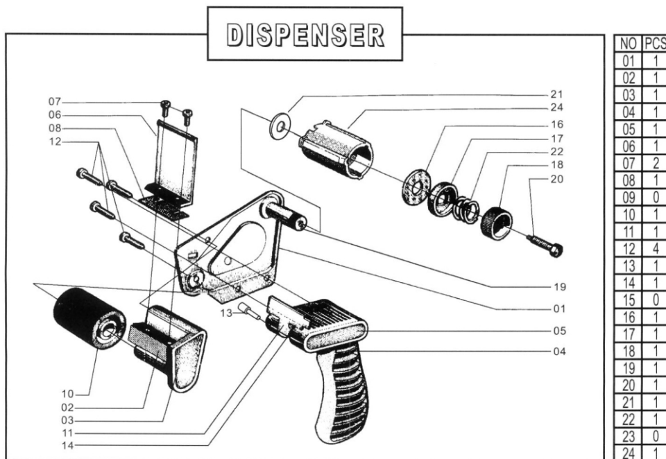
PEZZI DI RICAMBIO - SPARE PARTS LIST - LISTE DES PIECES DETACHEES - ERSATZTEILLISTE - LISTA DE REPUESTOS
