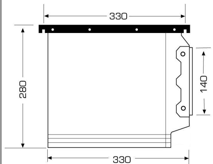
Schema Prodotto
